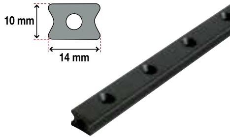
14 Schienen aus schwarz eloxiertem Aluminium, Serie 14 Für Grossschotschlitten
