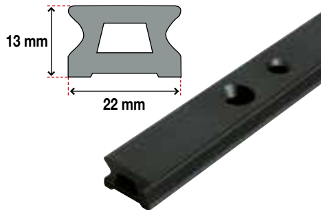
22 Schienen aus schwarz eloxiertem Aluminium, Serie 22 Für Grossschot- und Fockschlitten
