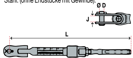
T10 Wantenspanner zum Abpressen, mit Graduierung Mit Gelenkgabel und Graduierung, aus rostfreiem Stahl. (ohne Endstücke mit Gewinde).
