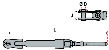
T10 Wantenspanner zum Abpressen Mit Gelenkgabel, aus rostfreiem Stahl. (ohne Endstücke mit Gewinde)
