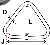
Dreieck Aus rostfreiem Stahl
