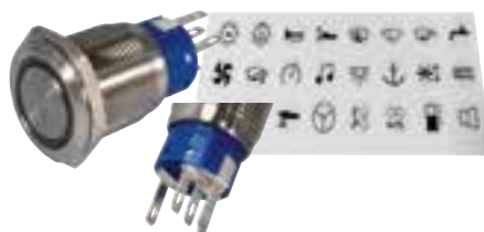
Schalter und Druckschalter mit LED 12 V, max 5 A. LED Beleuchtungsanschliessbar für Schalter oder Funktion. Masse: Ø 19 mm, Länge 33 mm
