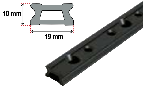
19 Schienen aus schwarz eloxiertem Aluminium, Serie 19 Für Grossschot- und Fockschlitten
