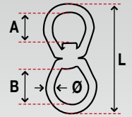
Wirbel (bei permanentem Eintauchen zu verwenden) Aus geschmiedetem rostfreien Stahl HR 17-4PH
