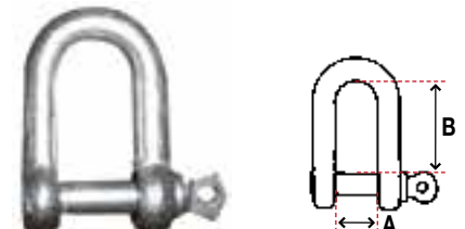
Gerade Schäkel Aus galvanisiertem Stahl
